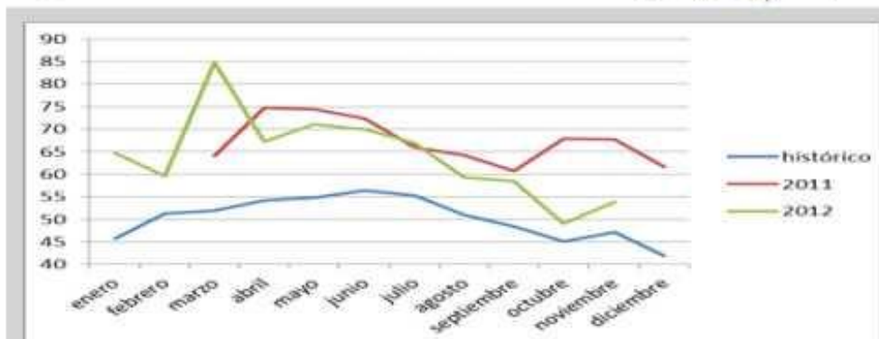
En la figura 2, analizamos la variación de la Corriente en el núcleo (máxima velocidad a 200 m de profundidad) en dicho correntómetro, ubicado casi al inicio de la Corriente Cromwell durante los años 2011 y 2012, comparado con la variación histórica mensual del promedio. Se puede observar claramente que en ambos años, su velocidad ha sido muy por encima de sus valores normales (entre un 30% a un 50% más rápida), lo que implica que esa intensificación ha incidido también en la zona cercana a Sudamérica y por consiguiente ha favorecido el retorno de las Merluzas de más edad a la zona de Perú.
