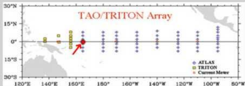
La Corriente Cromwell es registrada en varios correntómetros tal como se muestra en la Figura 1, resaltando en dicho gráfico con una flecha el correntómetro ubicado en los 0° N 165° E.
